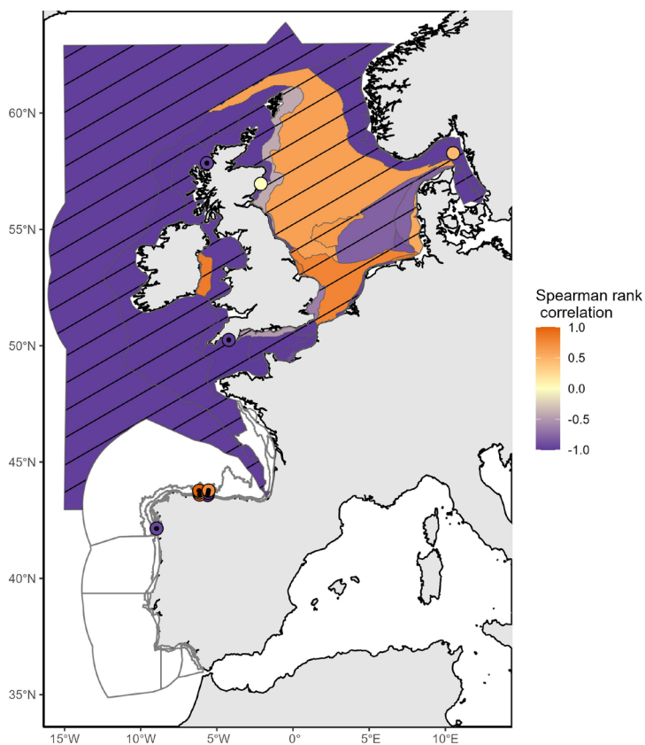
Figure 1 : Tendance des anomalies de la biomasse phytoplanctonique entre la période d'évaluation (2015-2019) et la période de comparaison (données des stations : 1992-2014 ; données des non-stations : 1997-2014). Les zones hachurées sont caractérisées par des changements significatifs ( p \leq 0,05 ) de la biomasse de phytoplancton entre la période de comparaison et la période d'évaluation. Les zones blanches indiquent l'absence de données ou des données insuffisantes pour évaluer la zone.
