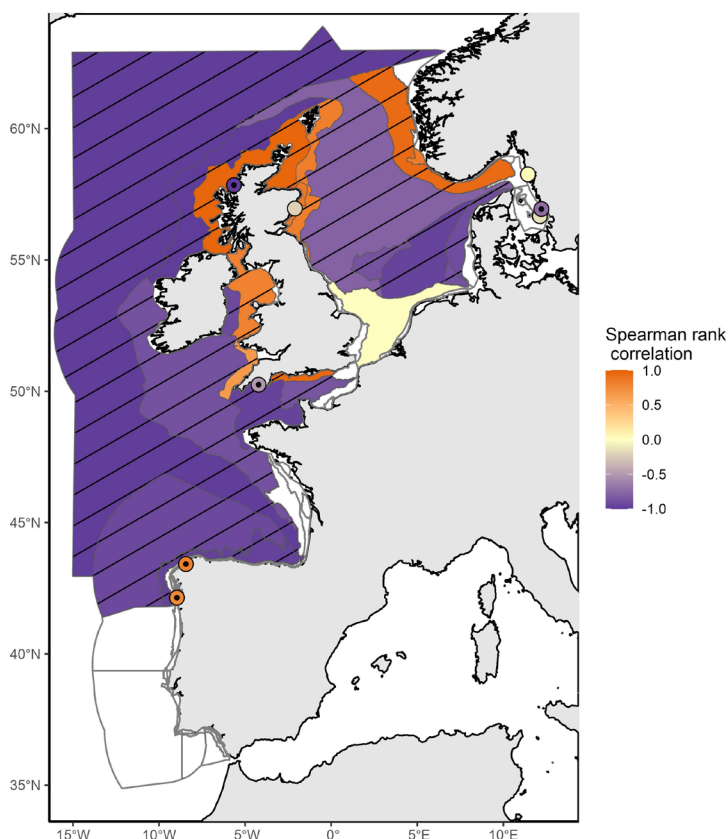
Figure 2 : Tendence des anomalies de l'abondance zooplanctonique entre la période d'évaluation (2015-2019) et la période de comparaison 1960-2014). Les zones hachurées sont caractérisées par des changements significatifs ( p \leq 0,05 ) de l'abondance zooplanctonique entre la période de comparaison et la période d'évaluation. Les zones blanches indiquent l'absence de données ou des données insuffisantes pour évaluer la zone. Les résultats des unités d'évaluation de la stratification intermittente 1 (Écosse) et de la stratification saisonnière de l'Atlantique (Irlande) doivent être interprétés avec prudence, car les échantillons du CPR ont été extrapolés sur des unités d'évaluation beaucoup plus vastes.
